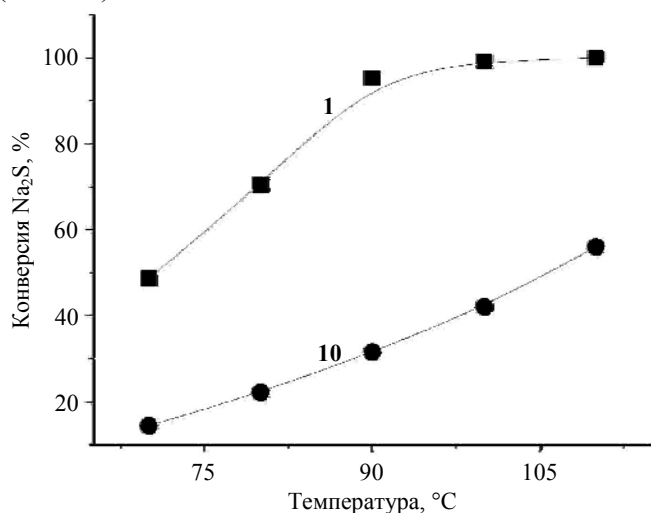
Рис. 4. Кинетические кривые окисления \text{Na}_2\text{S} стильбенхиноном 1 и дифенохиноном 10 ( [\text{Na}_2\text{S}]_0 0.09 моль/л, [\text{хинон}]_0 0.14 моль/л, 90 мин).
